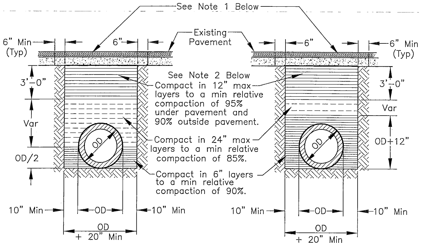
RIGID CONDUIT
